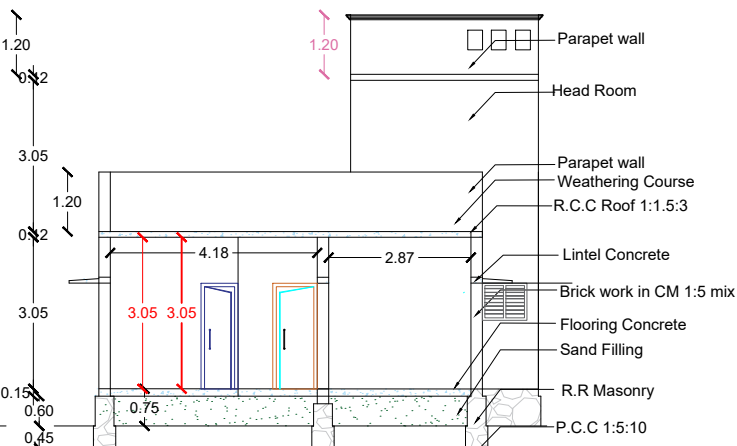
SECTION-E1E1
