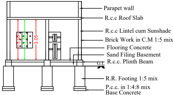
SECTION A-B
