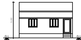
ELEVATION - 1
