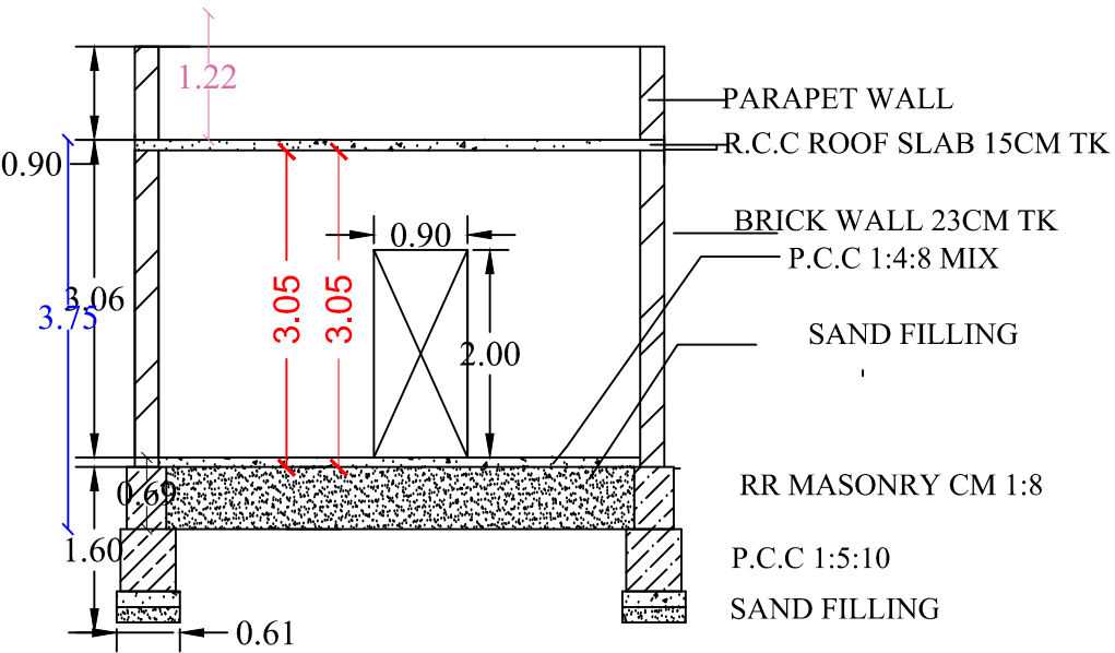
SECTION -AB
