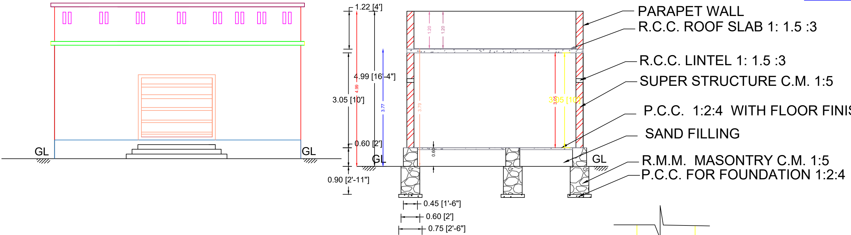
ELEVATION
