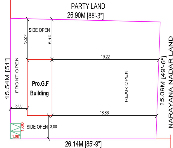
SITE PLAN (SCALE 1:200)
