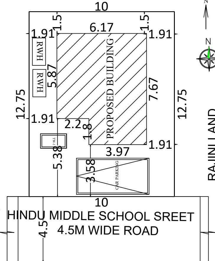
SITE PLAN 1:100 SCALE
