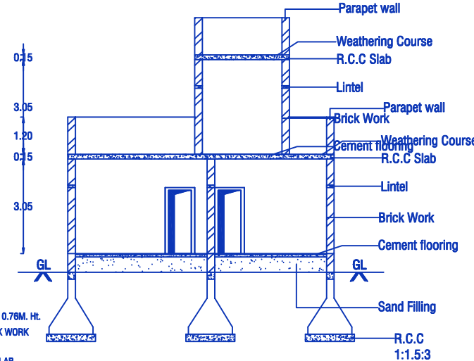
SECTION ON'AB'
