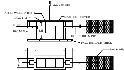
SECTION - AB
