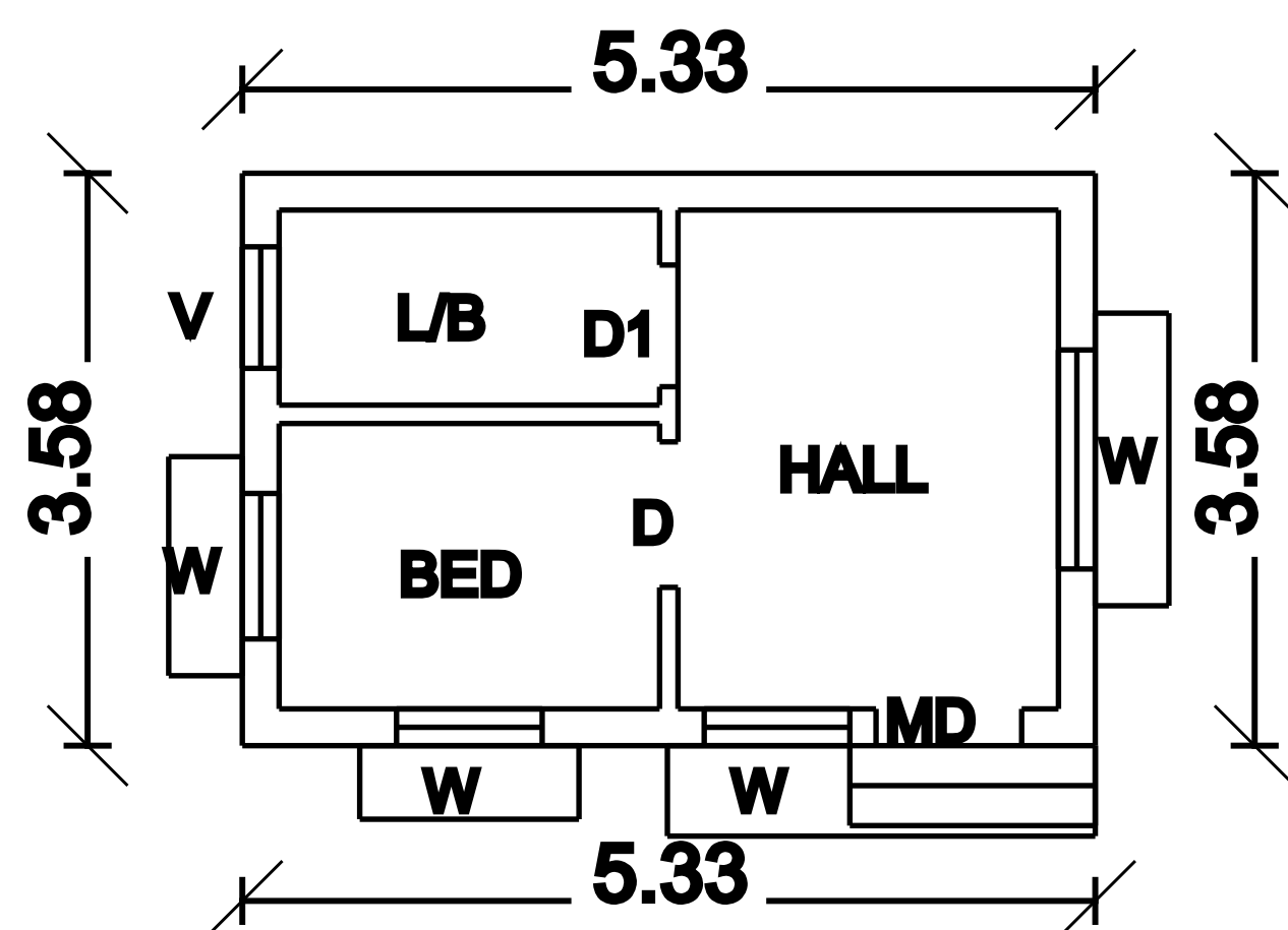
G.F PLAN
