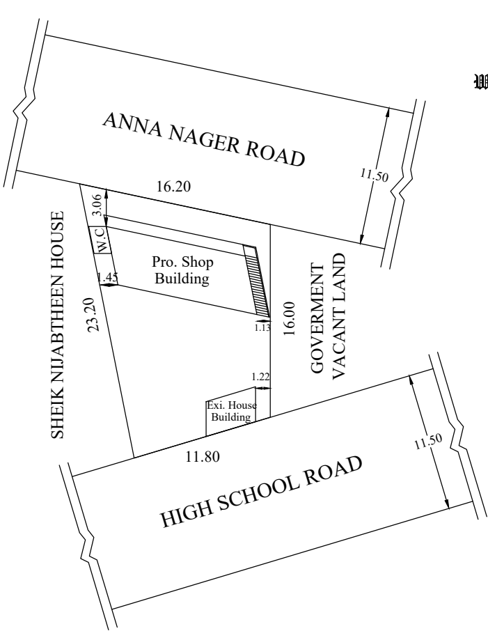
SITE PLAN SCALE 1:400
