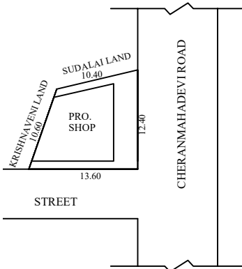
SITE PLAN SCALE 1:400
