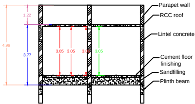
SECTION - AB
