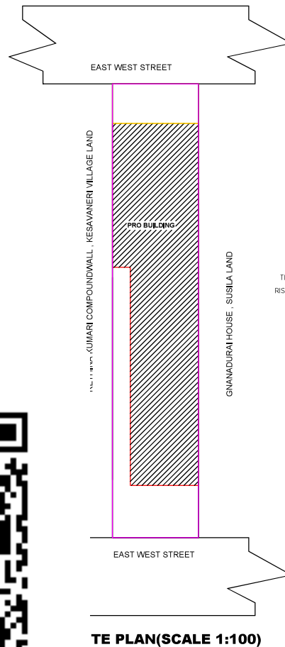
TE PLAN(SCALE 1:100)
