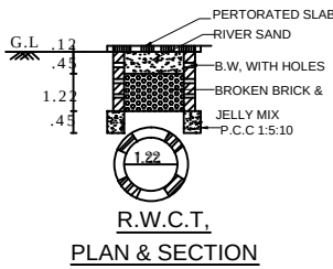
R.W.C.T. PLAN & SECTION
