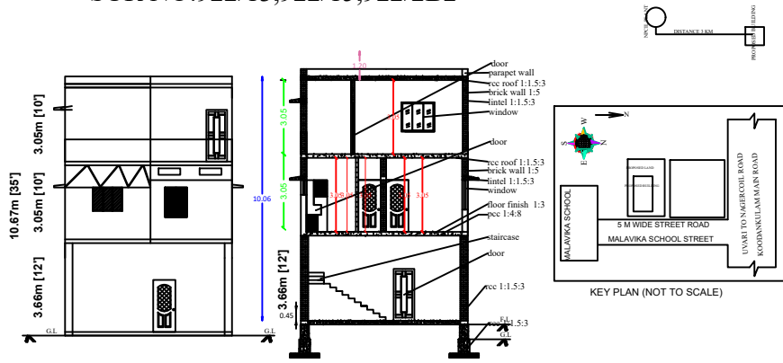
ELEVATION
