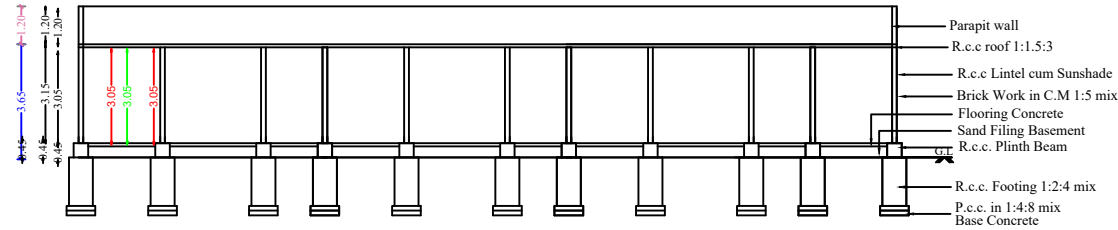
SECTION A-A
