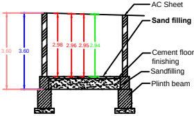
SECTION - AB
