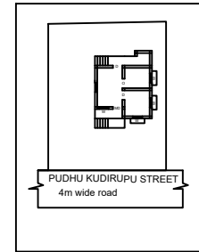
SITE PLAN 1:5 SCALE
