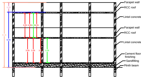
SECTION - AB
