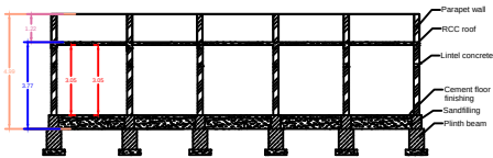
SECTION - AB
