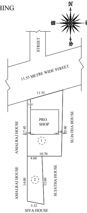
SITE PLAN SCALE 1:400
