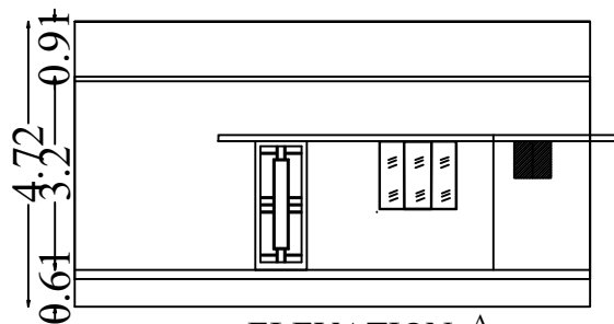
ELEVATION A-A
