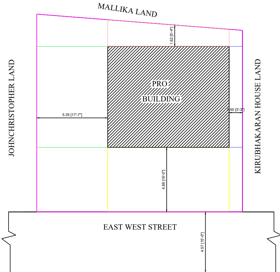
SITE PLAN(SCALE 1:100)
