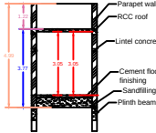
SECTION - AB
