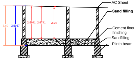
SECTION - AB
