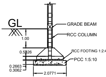
SECTION ON - BB (N.T.S)
