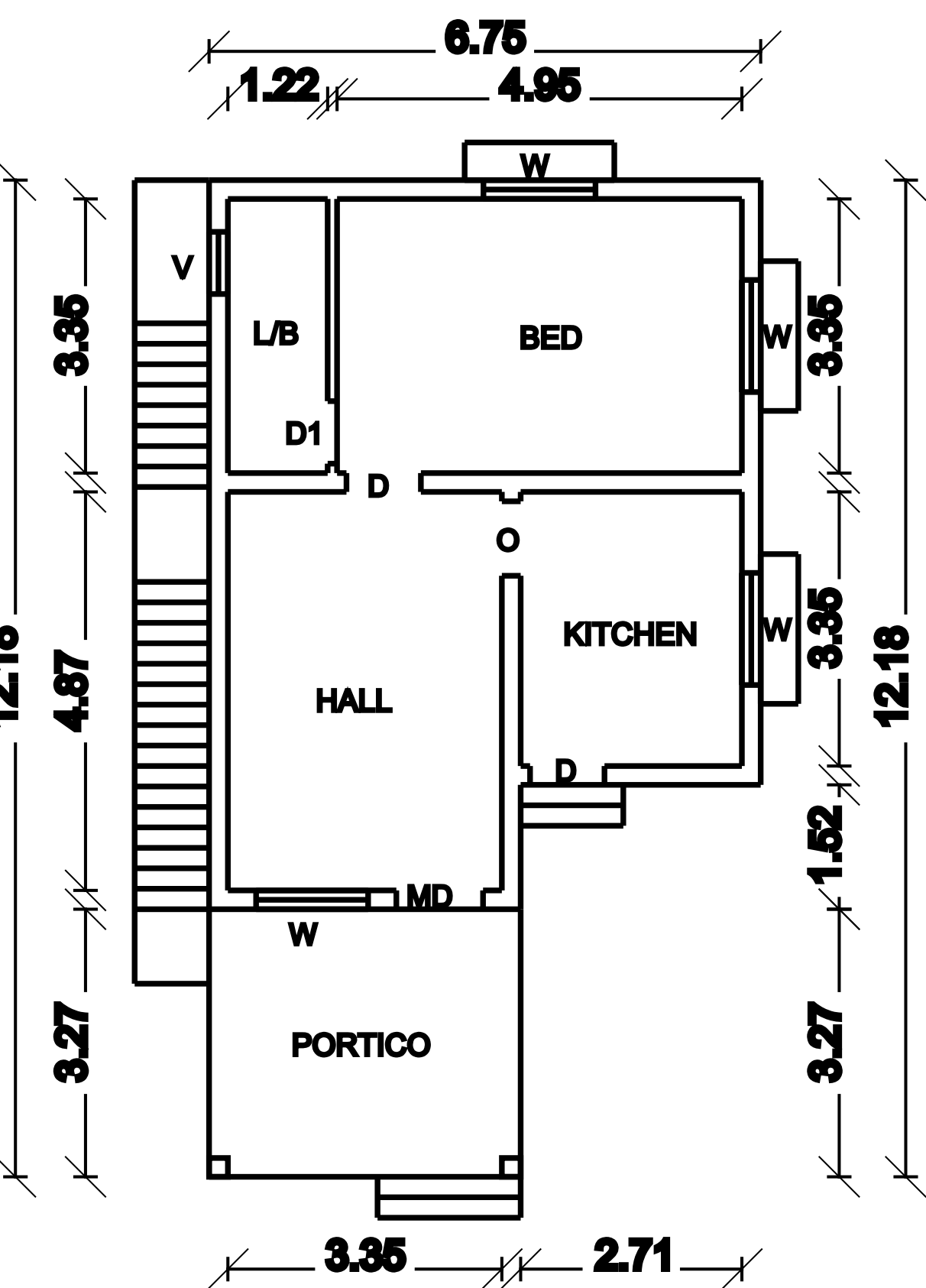
G.F PLAN
