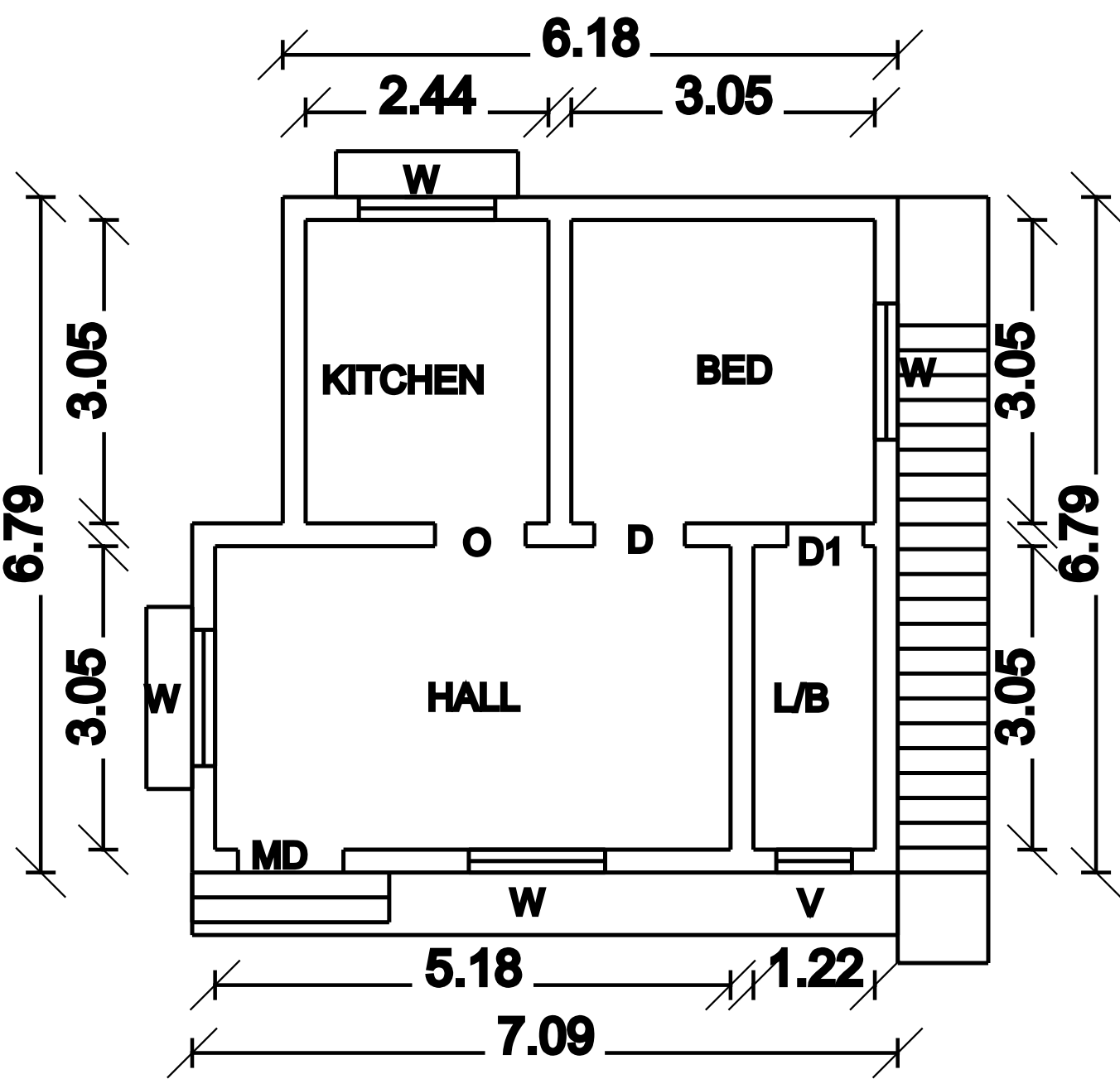
G.F PLAN
