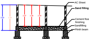
SECTION - AB
