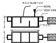
SEPTIC TANK AND TRENCH N.T.S
