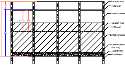
SECTION - AB
