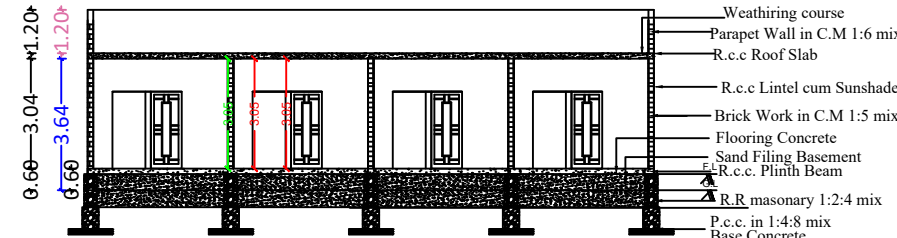
SECTION A-B
