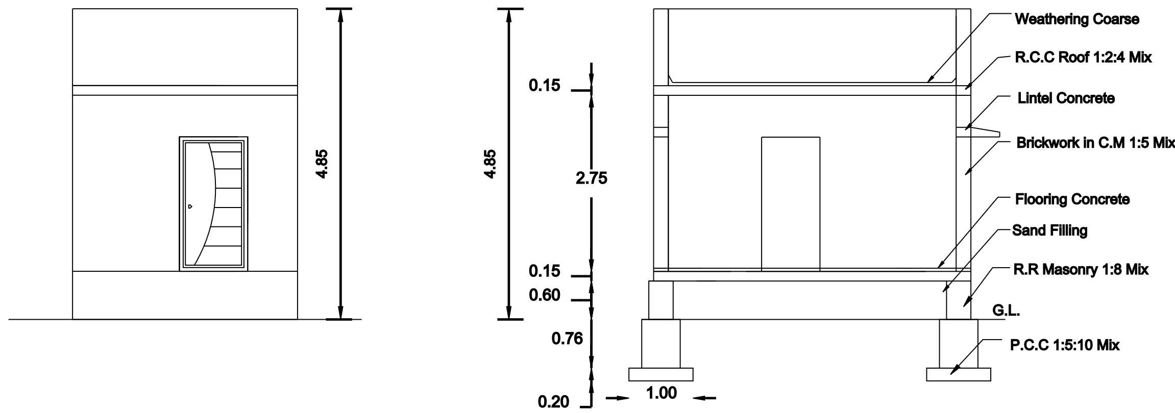
ELEVATION
