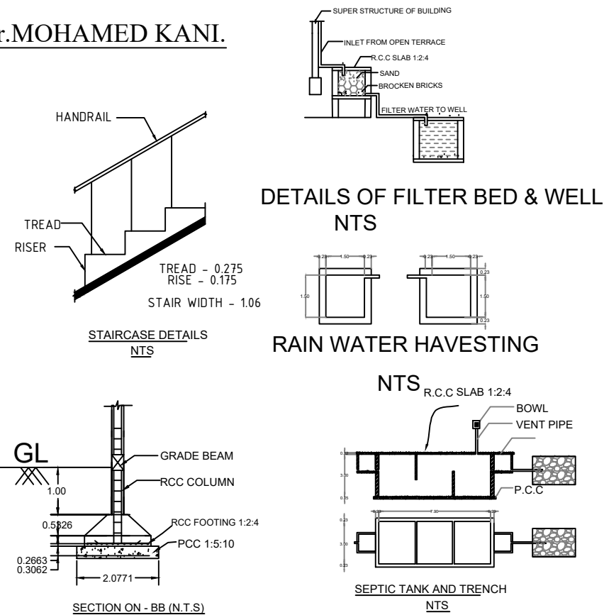
SECTION ON - BB (N.T.S)
