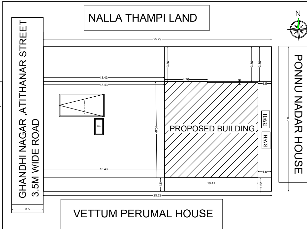
SITE PLAN 1:100 SCALE
