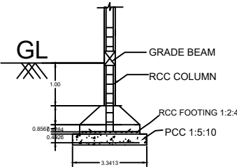
SECTION ON - BB (N.T.S.)
