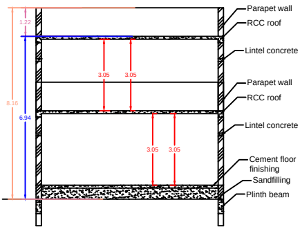
SECTION - AB
