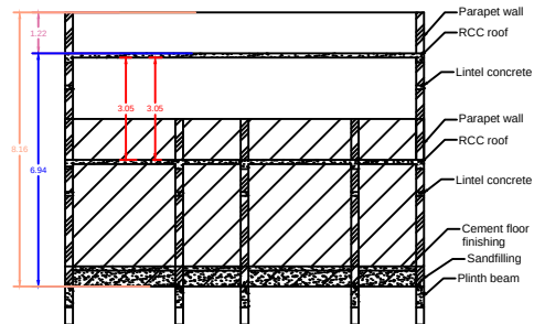
SECTION - AB
