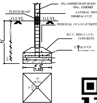
FOUNDATION DET.
