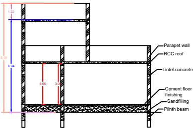
SECTION - AB
