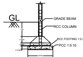
SECTION ON - BB (N.T.S)
