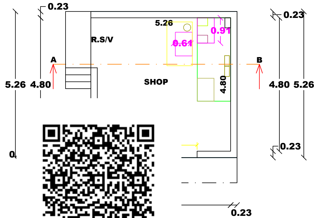
DR PLAN
