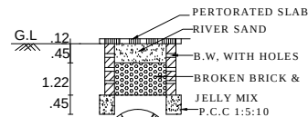
R.W.C.T. PLAN & SECTION
