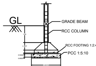
SECTION ON - BB (N.T.S)
