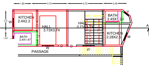
F.F.PLAN
