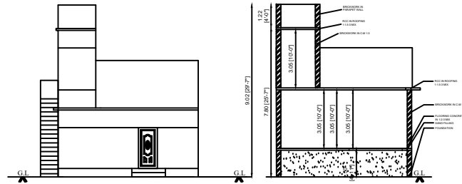
ELEVATION
