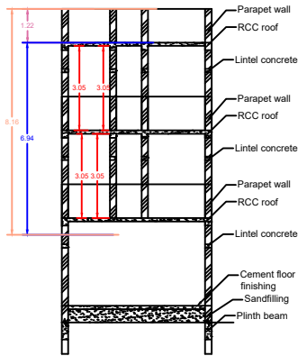
SECTION - AB
