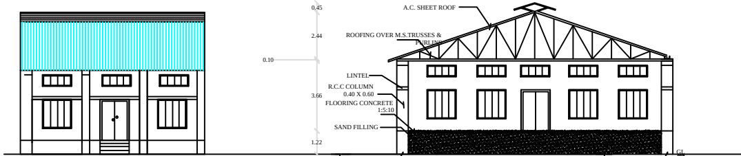
ELEVATION
