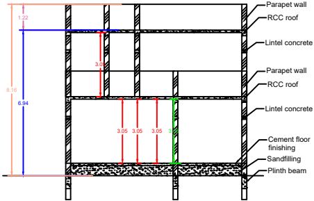
SECTION - AB
