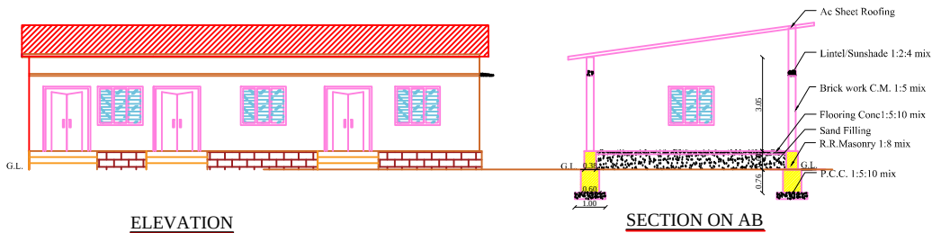
ELEVATION
